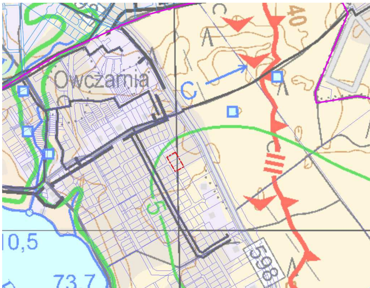
Ryc.5. Położenie obszaru opracowania na tle mapy hydrograficznej
