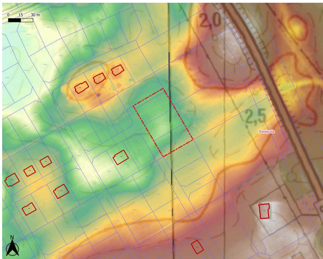
Ryc.4 Obszar projektu planu – rzeźba terenu.
